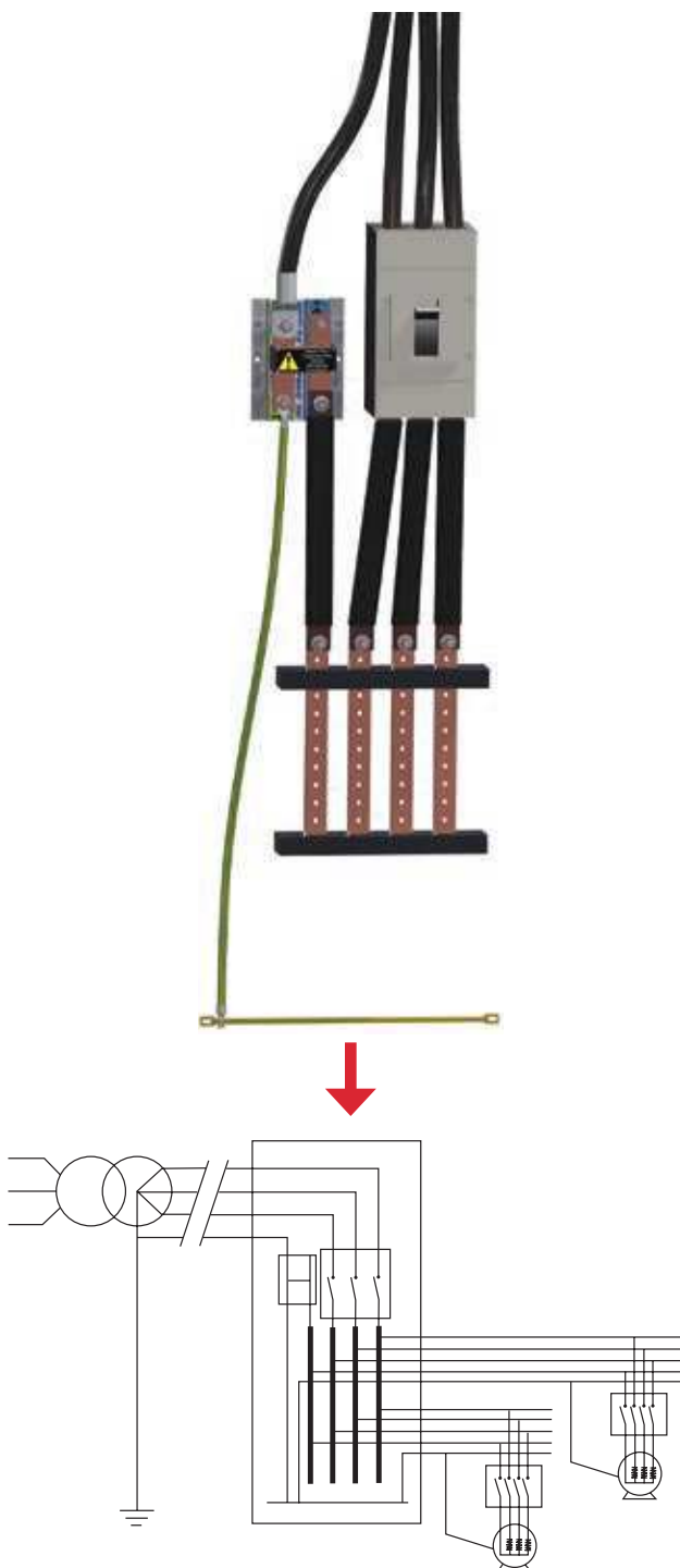
TN-S分线
