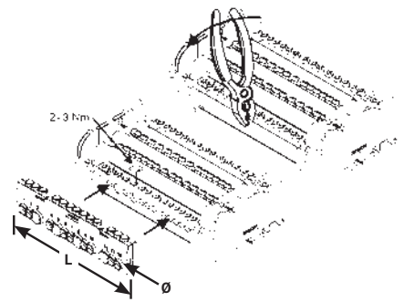
安装中性排示意
